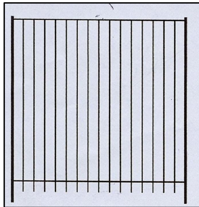
DECORATIVE FENCE ELEVATION SCALE: N.T.S.
